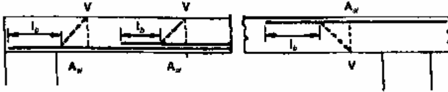
Fig - 3-1 per l_b lunghezza di ancoraggio, vedasi punto 5.3.3.
