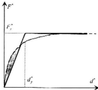
Figura 4.1 - Diagramma bilineare equivalente
