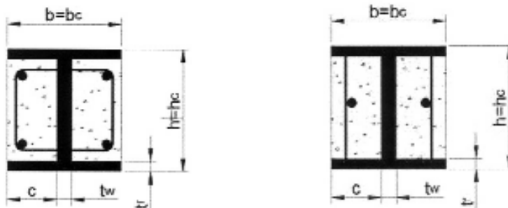
a) Staffe saldate all'anima
