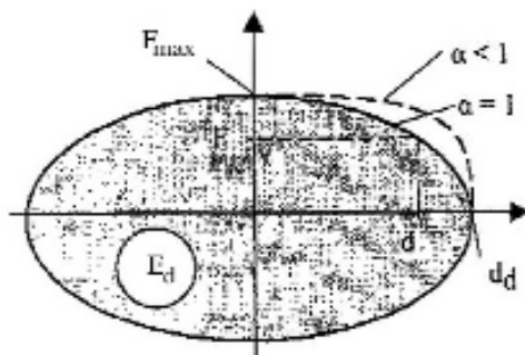
Figura 10.2 - Dispositivi a comportamento viscoso
