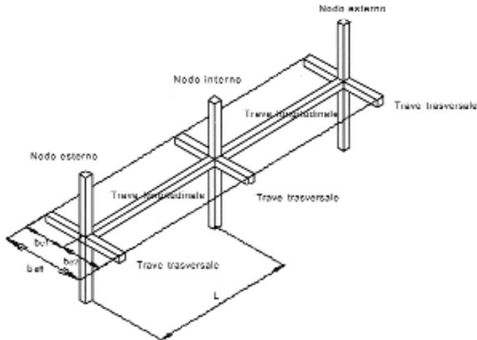
Figura 7.5 - Definizione degli elementi in una struttura intelaiata
