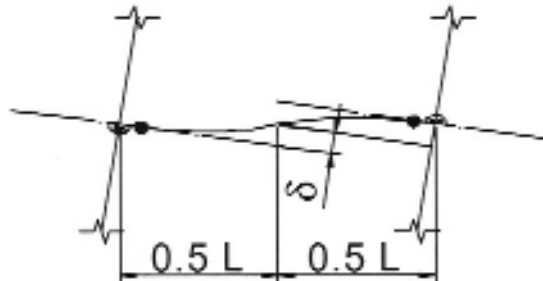
Figura 7.7 - Calcolo della capacità di rotazione plastica
