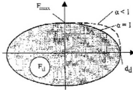
Figura 2 - Dispositivi a comportamento viscoso
