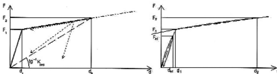
Figura 10.1 - Diagrammi forza-spostamento per dispositivi non lineari
